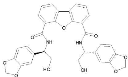
20 (CDCl 3 , 500 MHz)
