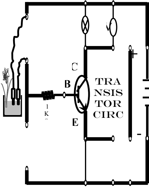
شكل (46): الري الأتوماتيكي
