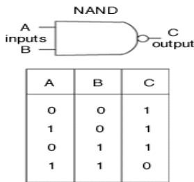
شكل (47) : بوابة NAND
