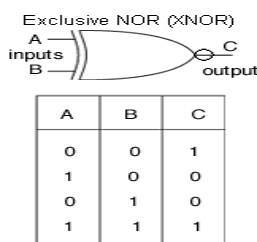
شكل (50) : بوابة XNOR
