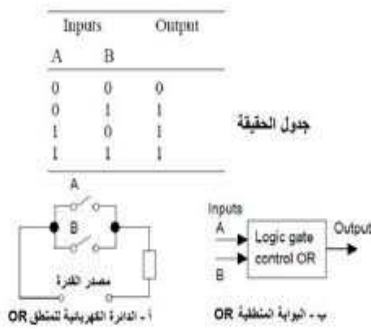
الشكل ٤٠: يبين البوابة المنطقية OR
