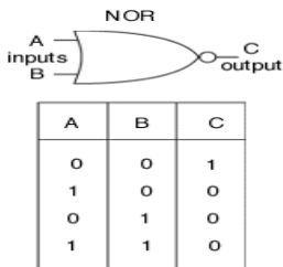
شكل (48) : بوابة NOR
