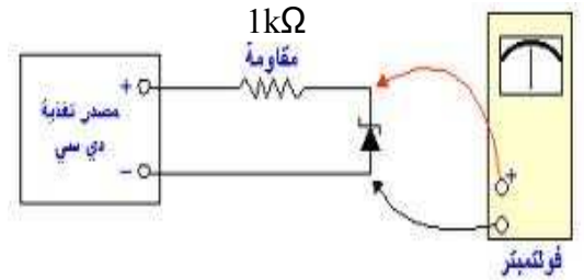
شكل (21): اختبار جهد ثنائي الزينر
