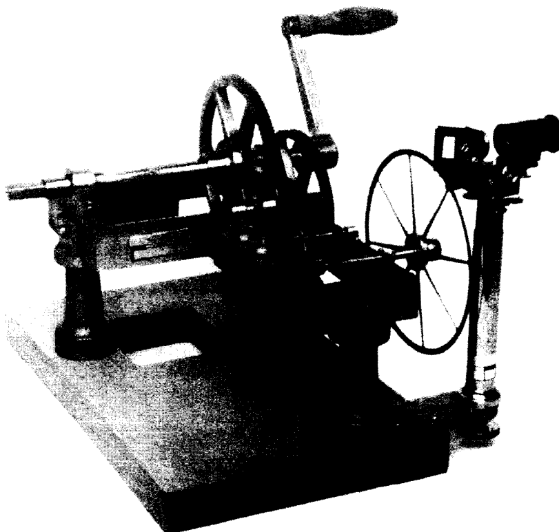
Fig. 28. Fizeau's Machine
