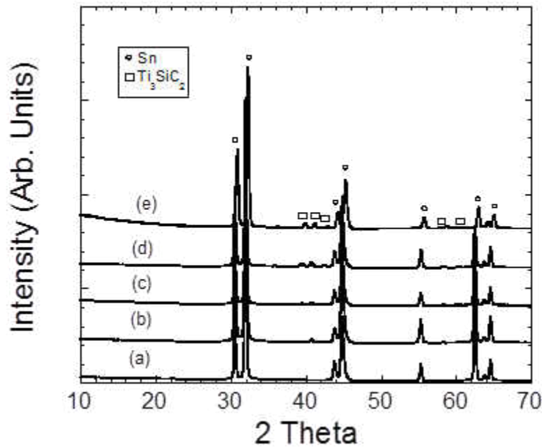
Figure 3.1. XRD profiles of, (a) Sn, (b) Sn(95)- \text{Ti}_3\text{SiC}_2 (5), (c) Sn(90)- \text{Ti}_3\text{SiC}_2 (10), (d) Sn(80)- \text{Ti}_3\text{SiC}_2 (20), (e) Sn(70)- \text{Ti}_3\text{SiC}_2 (30).
