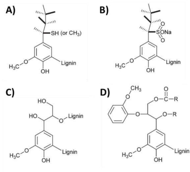
Figure 1. A) Kraft lignin, B) Lignosulfonate, C) Soda lignin, D) Organosolv lignin. (Kai et al., 2016)
