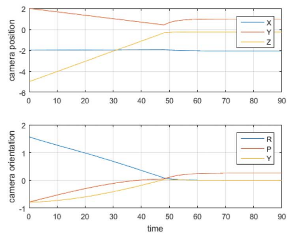
(d) ANN based Control
