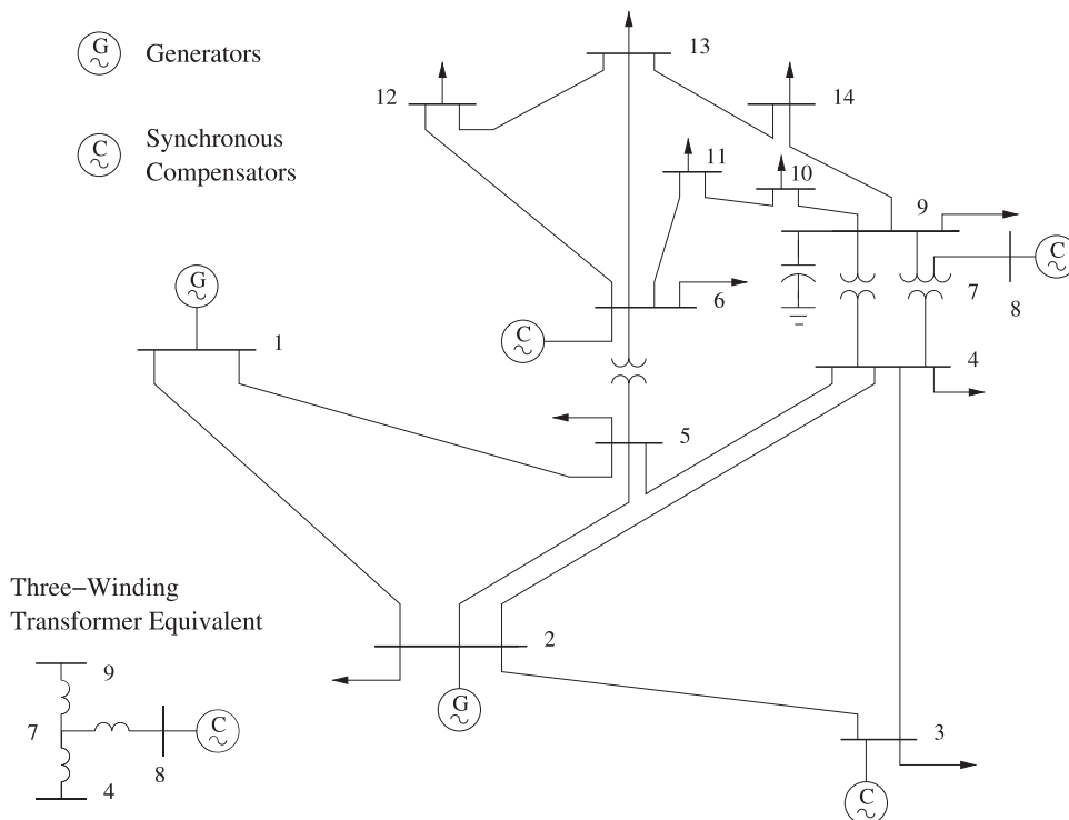
Fig. 5. IEEE 14-bus system.
