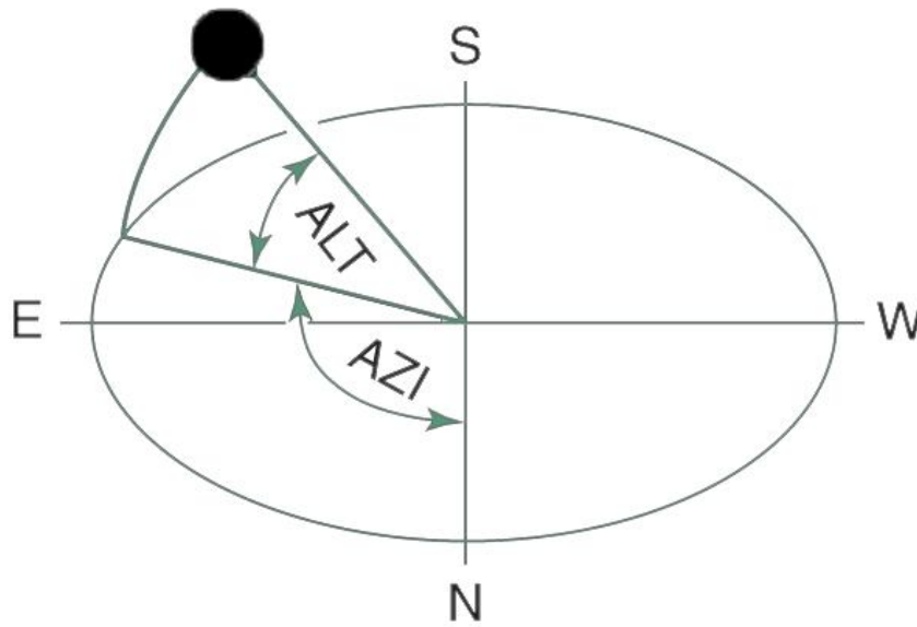
Fig. 3.11 : Altitude and azimuth angles
