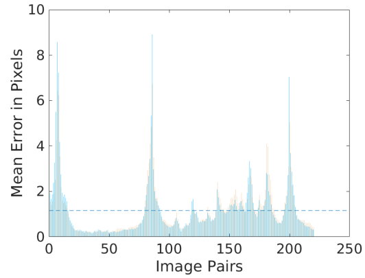
(d) Filtered underwater dataset with SuperView
