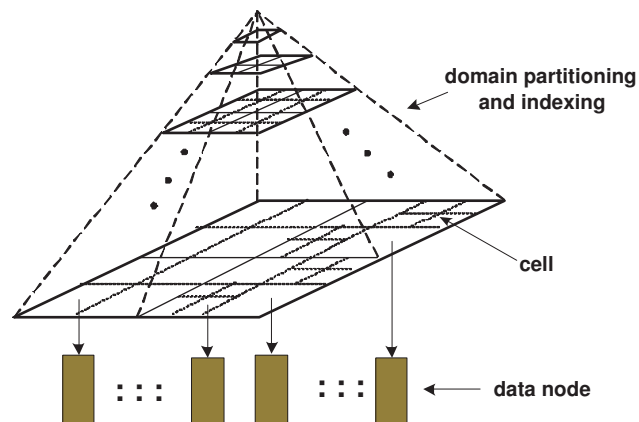
Figure 3.1 POI indexing
