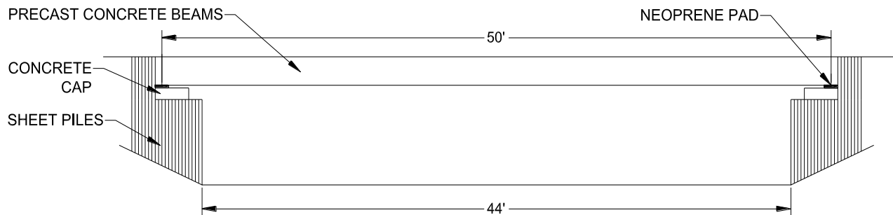
b. Elevation
