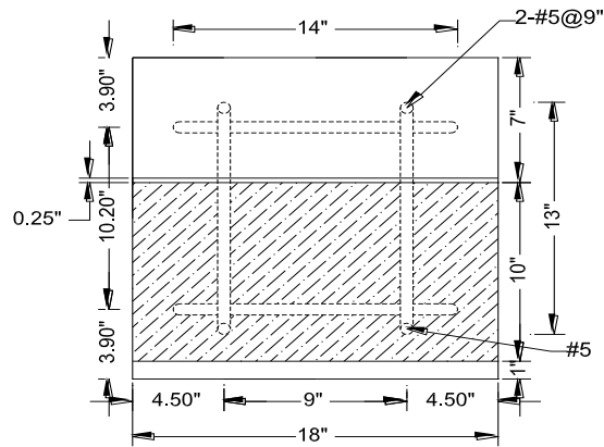
c) SECTION B-B'
