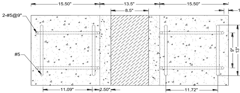
b) SECTION A-A'
