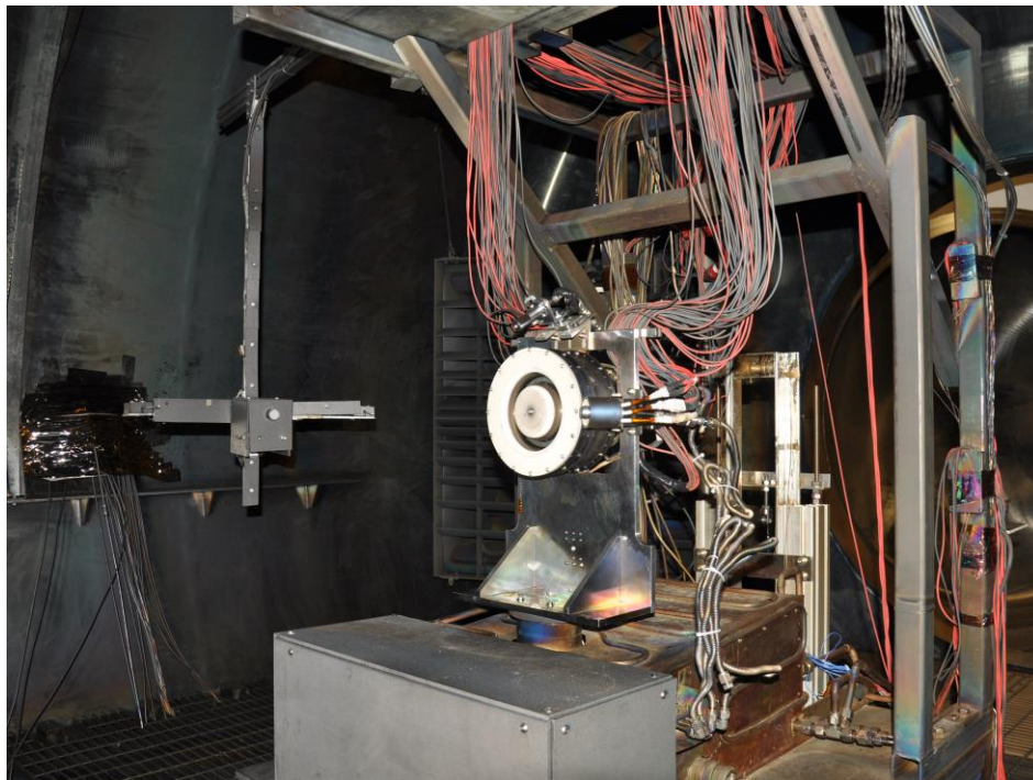
Figure 4.2: IHD2000-EM11 HET installed in VTF-2.
