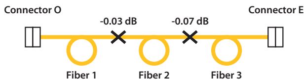
Actual fusion splice loss
