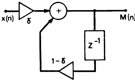
FIG. 3.3 Recursive estimator.
