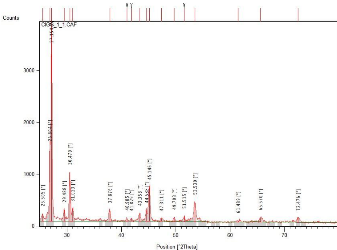
Fig. 4.4. XRD for CZSS 50.
