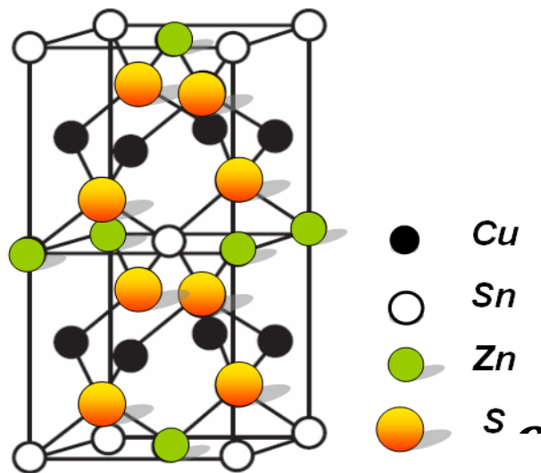
Fig. 2.17. CZSS structure. [23]
