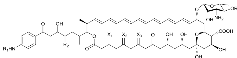
mycoheptin 155
