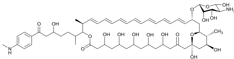
perimycin A 162
