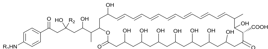
perimycin A 162
