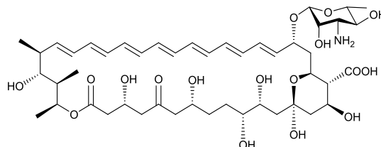
mycoheptin 155
