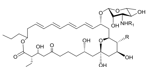
rimocidin 10 R = COOH rimocidin B 11 R = CONH 2 rimocidin C 12 R = CH 3
