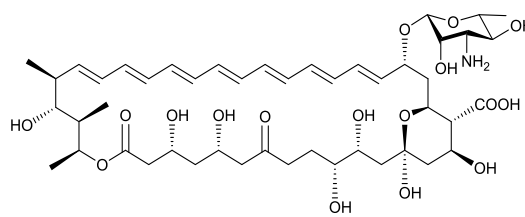
candicidin 154
