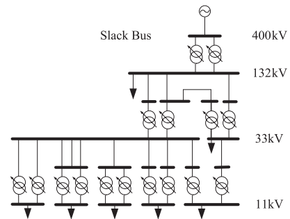
Fig. 10 UKGDS_A
