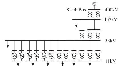
Fig. 12 UKGDS_C
