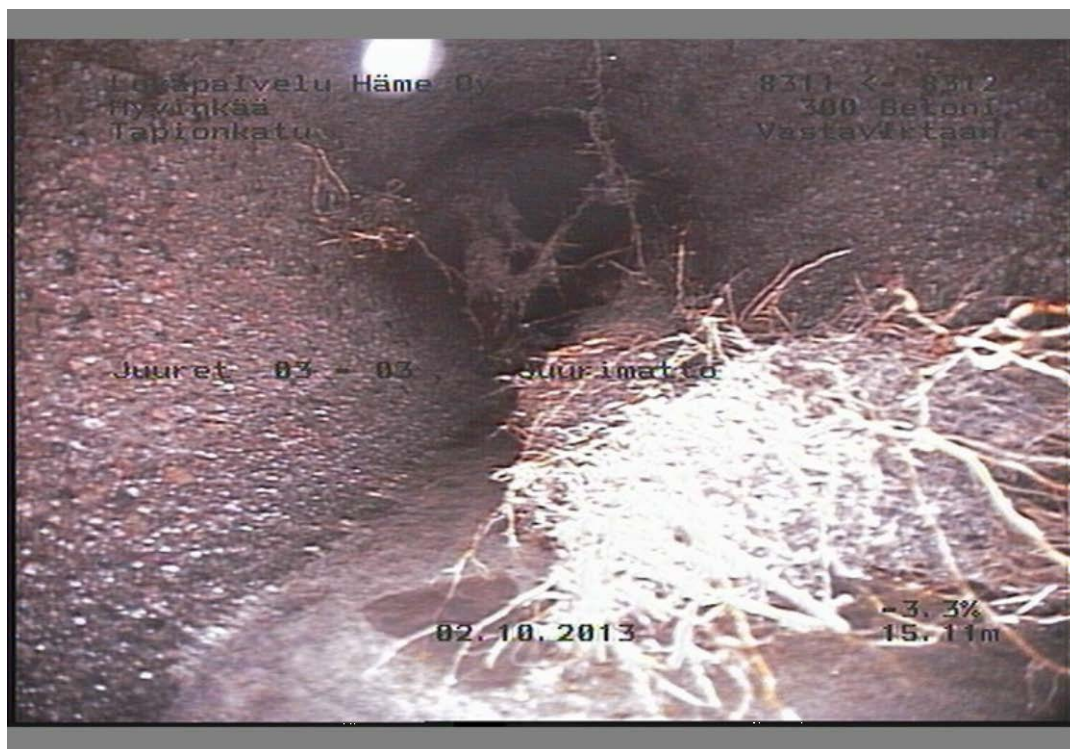
Kuva 6. Betoniputken sisään työntäviä puunjuuria. (Hyvinkään Vesi).
