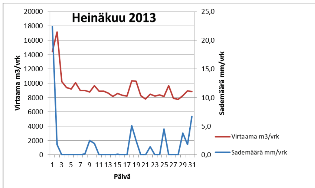
Kuva 9. Kaltevan jätevedenpuhdistamolle saapunut jätevesivirtaama ja sademäärät heinäkuussa vuonna 2013. Heinäkuun alussa rankkasateen aikana puhdistamon jälkiselkeyttimen ohi meni vettä 680 \text{ m}^3 .
