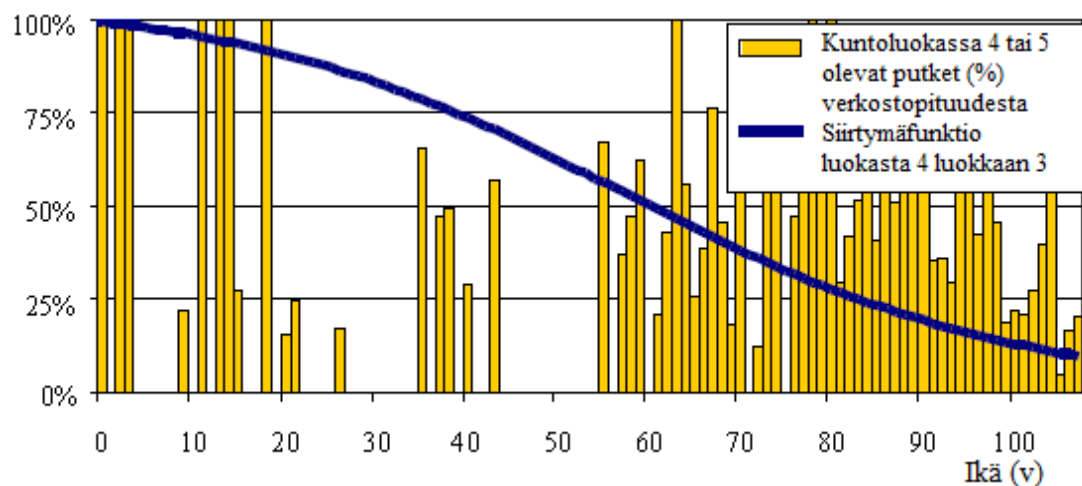
Kuva 8. Siirtymäfunktion, joka kuvaa putken siirtymistä kuntoluokasta 4 kuntoluokkaan 3. (mukaillen lähdettä Bauer ja Herz 2002).
