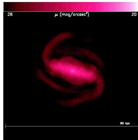
(b) nfw1 - 2.600 Gyr
