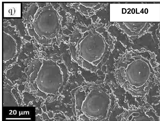
Figure 4-4 (Cont) SEM micrographs of the patterned samples m) D10L20, n) D10L30, o) D20L20, p) D20L30 and q) D20L40 after corrosion.
