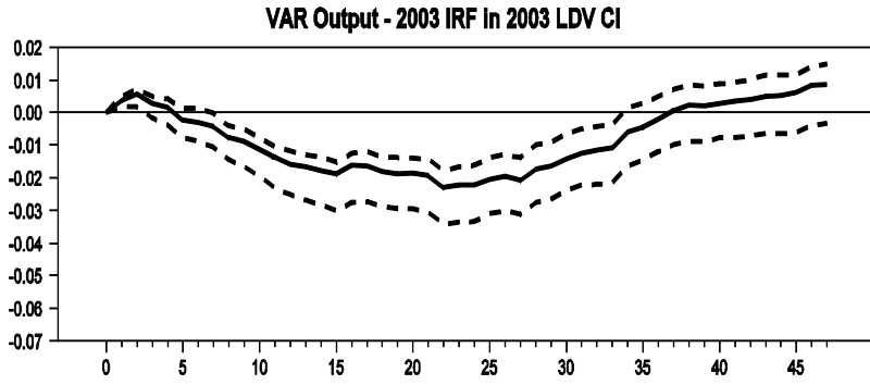
(fig. 2.5 cont'd.) e
