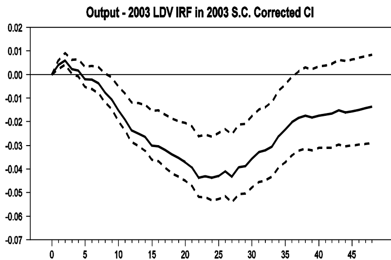
(fig. 2.3 cont'd) g
