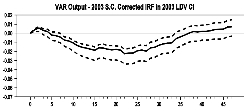
(fig. 2.5 cont'd.) f
