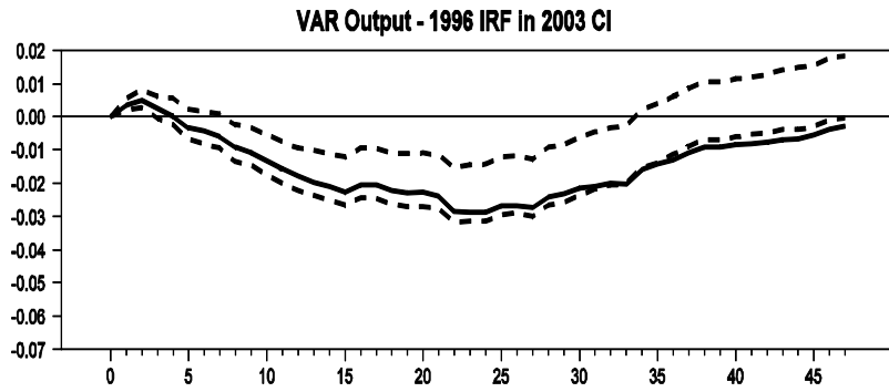
(fig. 2.5 cont'd.) b
