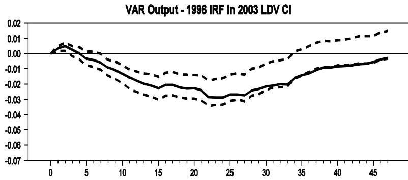
(fig. 2.5 cont'd.) d
