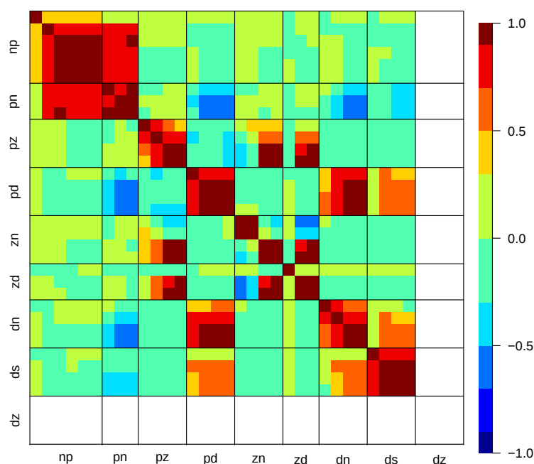
(a) OG99NPZD
