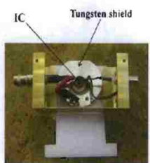
(d) AEFC internal components [19]
