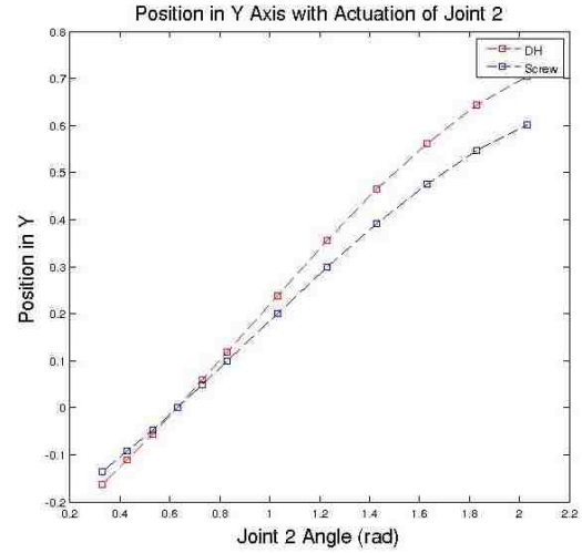
(b) Estimated and Actual Y position
