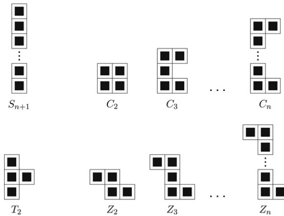
Fig. 4.1. The winner \mathcal{W}_n .
