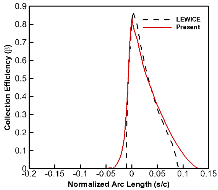
a) AoA = -1 deg.
